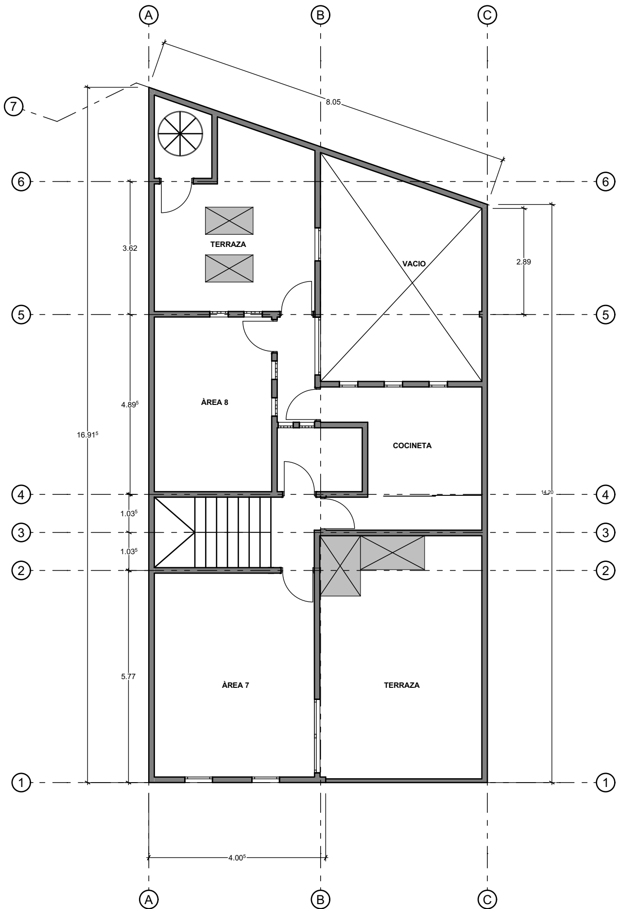
PLANTA SEGUNDO NIVEL
